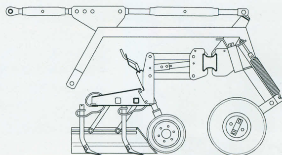
Roerækkerenser 6-rækket i indsats ved små roeplanter.
