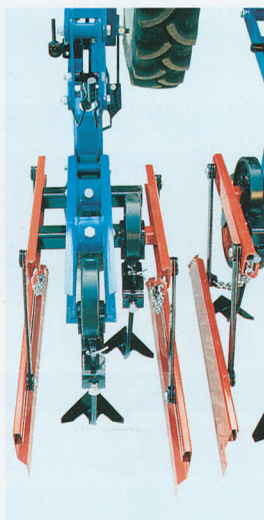
Roerækkerenser 6-rækket i indsats ved små roeplanter
