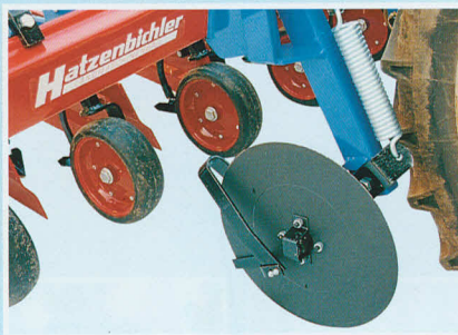
Hatzenbichler 4-rækket majsrækkerenser med automatisk styring, gødningsspreder og plantebeskyttelsesplader
